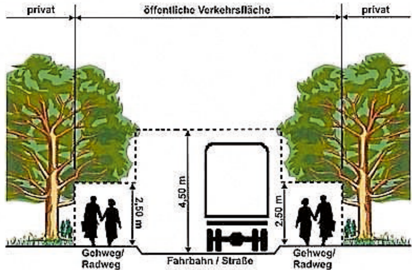
Lichtraumprofil an öffentlichen Straßen, Wegen und Plätzen
